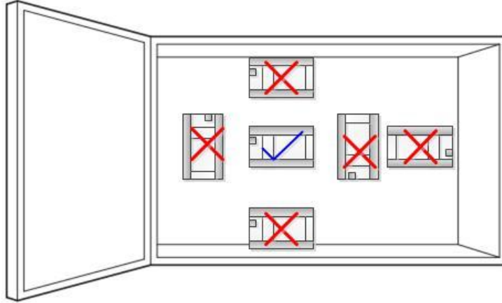
图 8-1 PLC在电柜中安装位置
