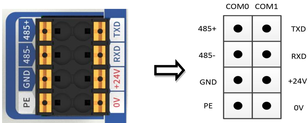
图 4-2 电源&amp;通讯端子引脚图
