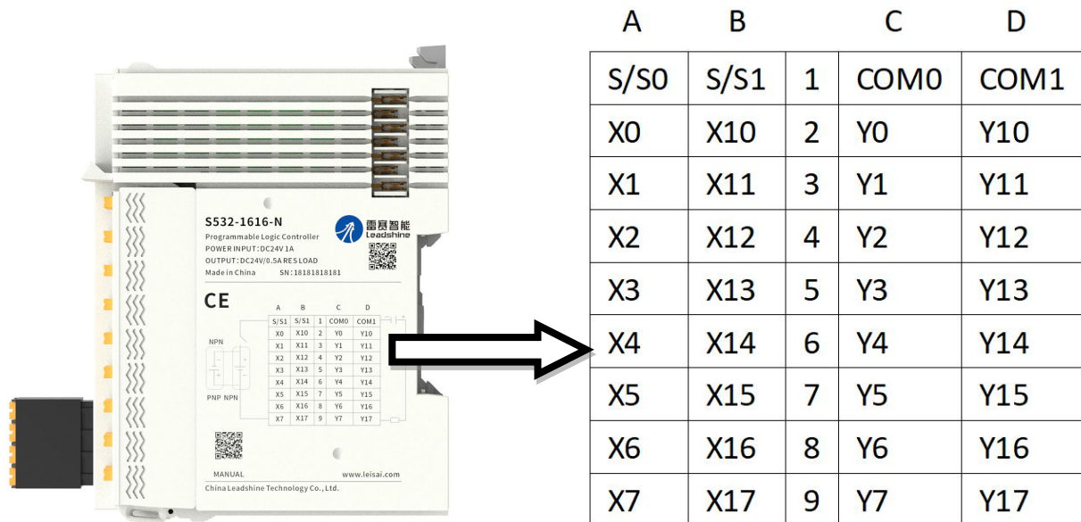
图 4-1 产品右侧端子丝印示意图
