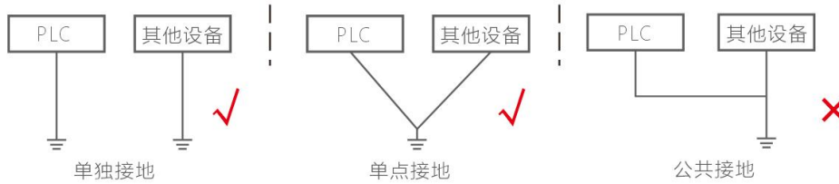
图 1-1 接地类型图
