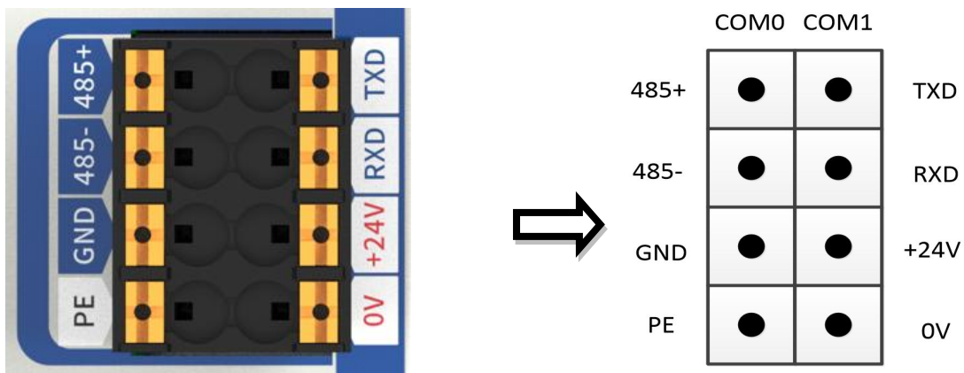
图 5-3 RS485 &amp; RS232通信端口示意图
