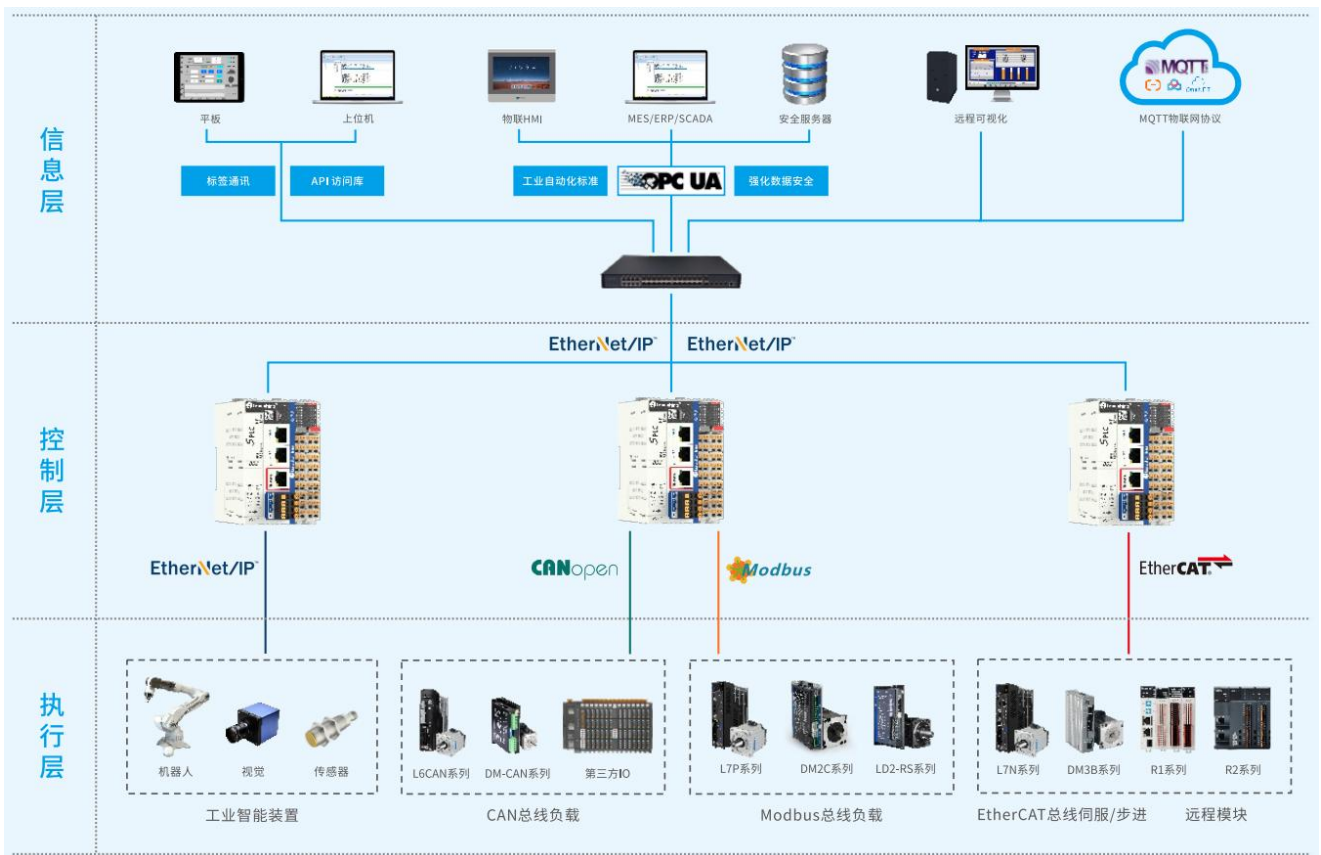
图 5-1 S6系列PLC组网拓扑图
