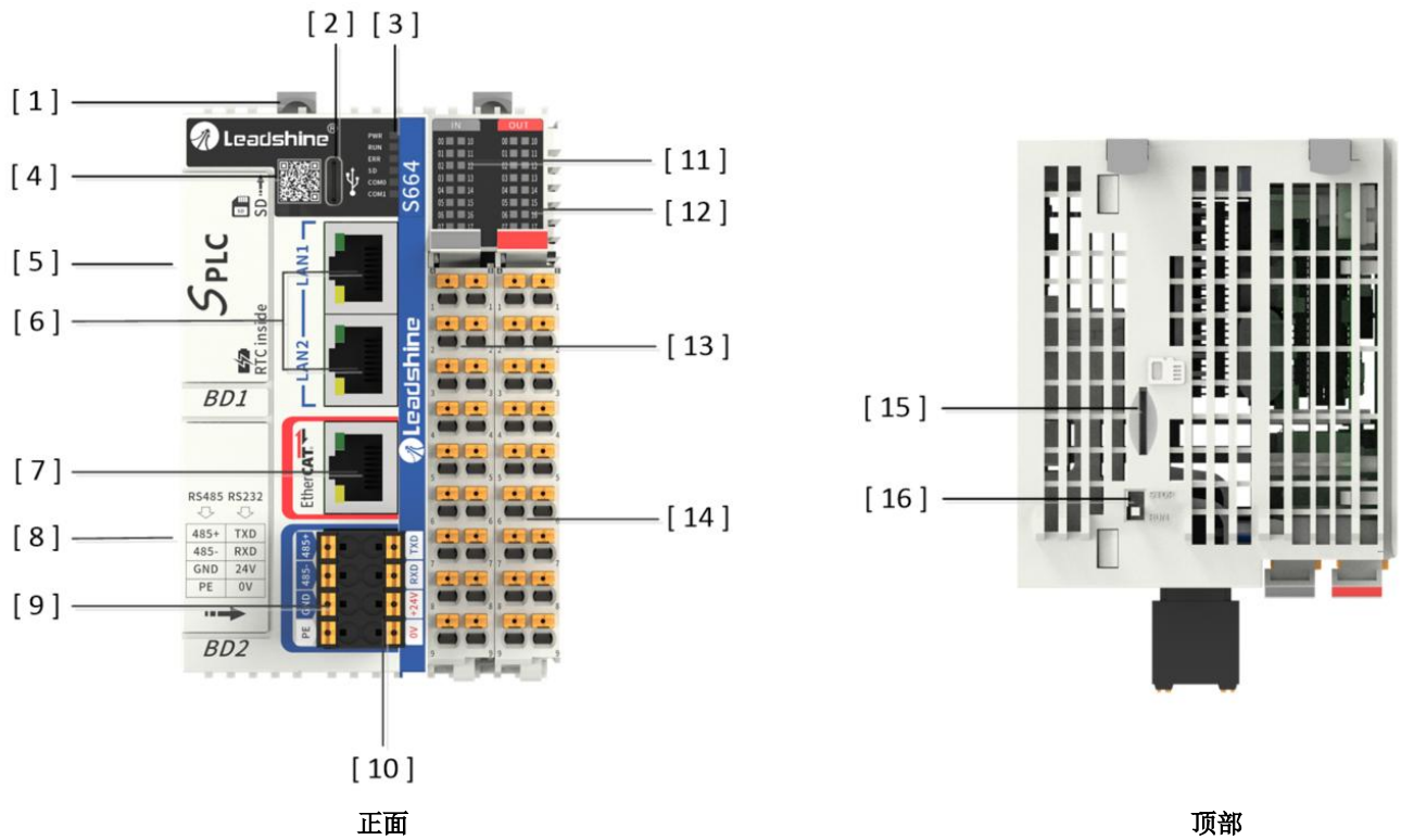
图 2-1 S6系列PLC正面外部接口图
