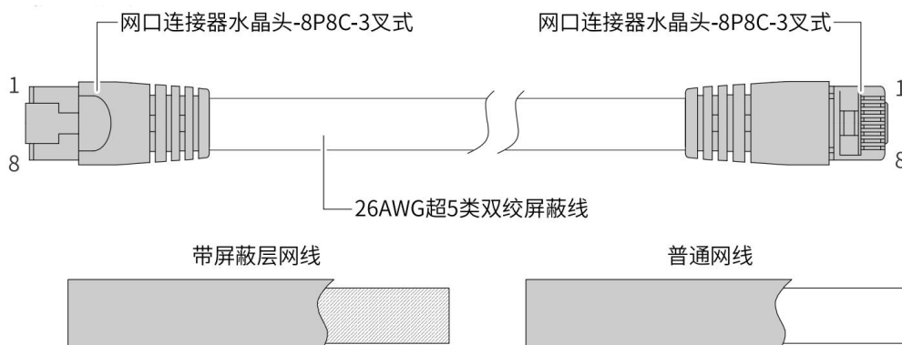
图 5-2 以太网线缆
